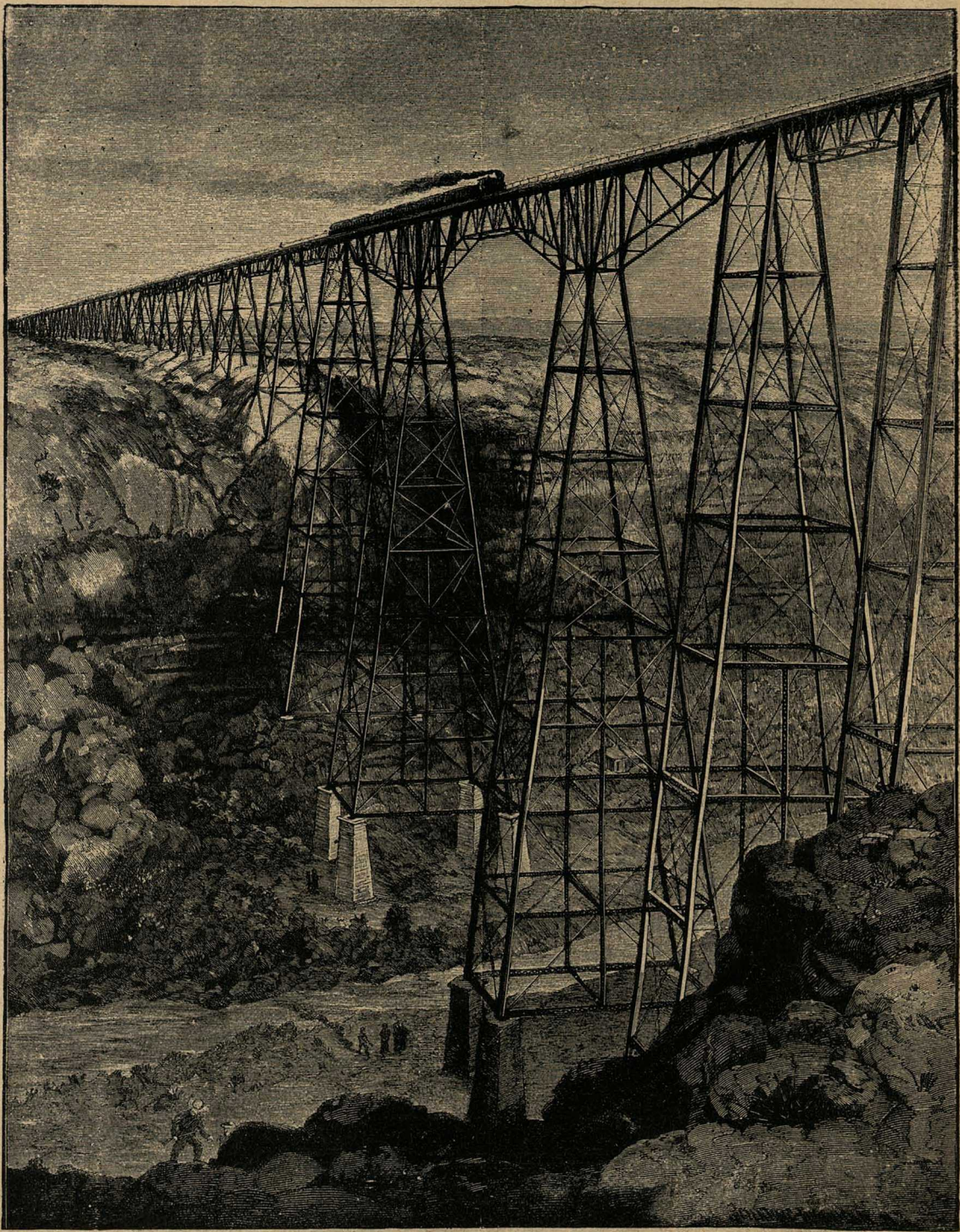
Мостъ на Тихо-океанской желѣзной дорогѣ въ Сѣверной Америкѣ.
